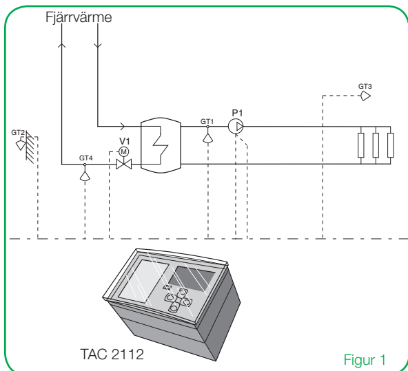
Fjärrvärmesystem
