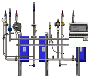
TP-XM-TRV Tappvarmvattenberedning och 2 värmekretsar
